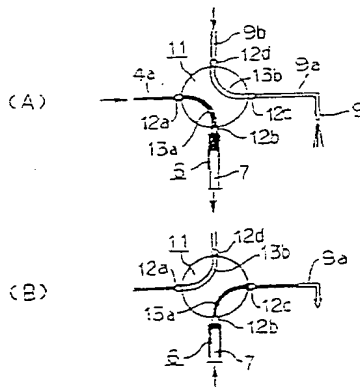
本発明の第二の実施の形態を示す流路図
